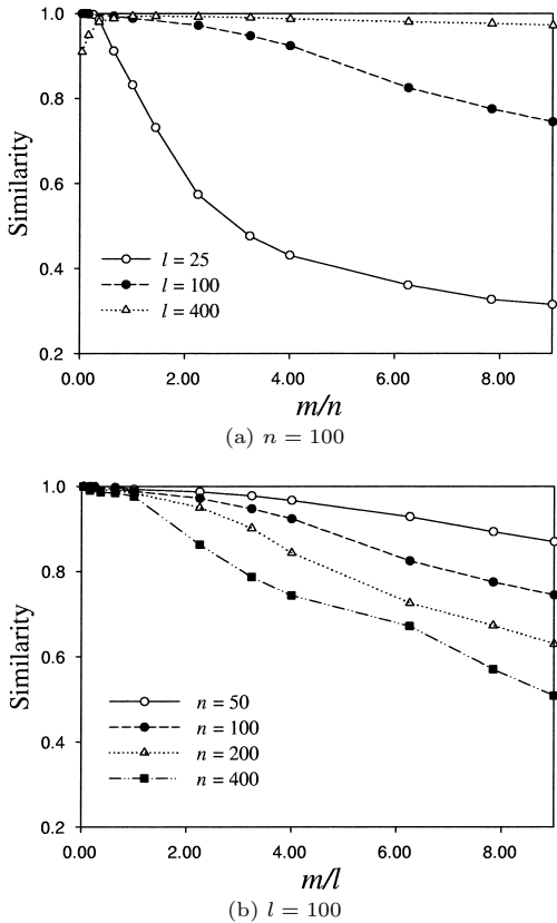
図2 BPモデルの学習性能
