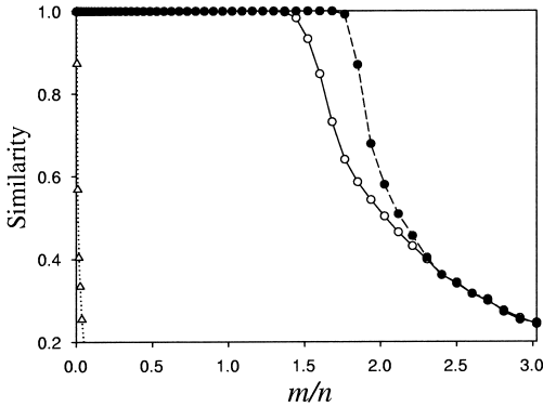
図 6 積型修飾モデルの学習容量
