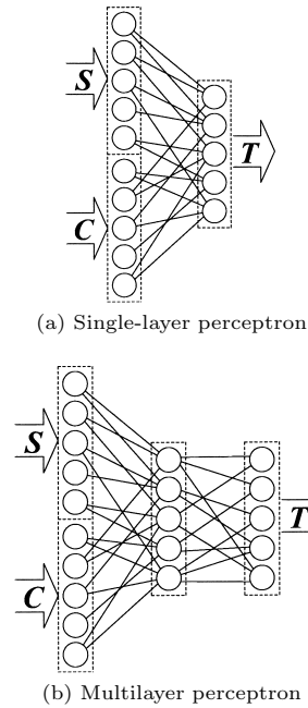
図 1 層状ニューラルネットの構造 Fig. 1 Architecture of layered neural networks.
